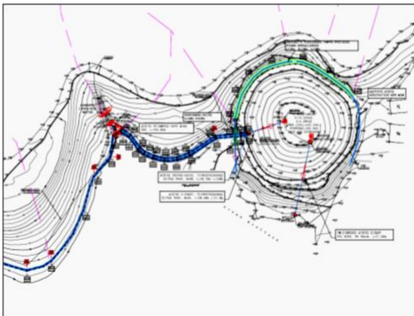
Σχέδιο 3 (απόδοση χωρίς κλίμακα) : Προτεινόμενη διαμόρφωση έργου (αγωγός προσαγωγής νερού από Χ.Θ.: 0+453 έως Χ.Θ.: 0+685 και Λιμνοδεξαμενή ).
