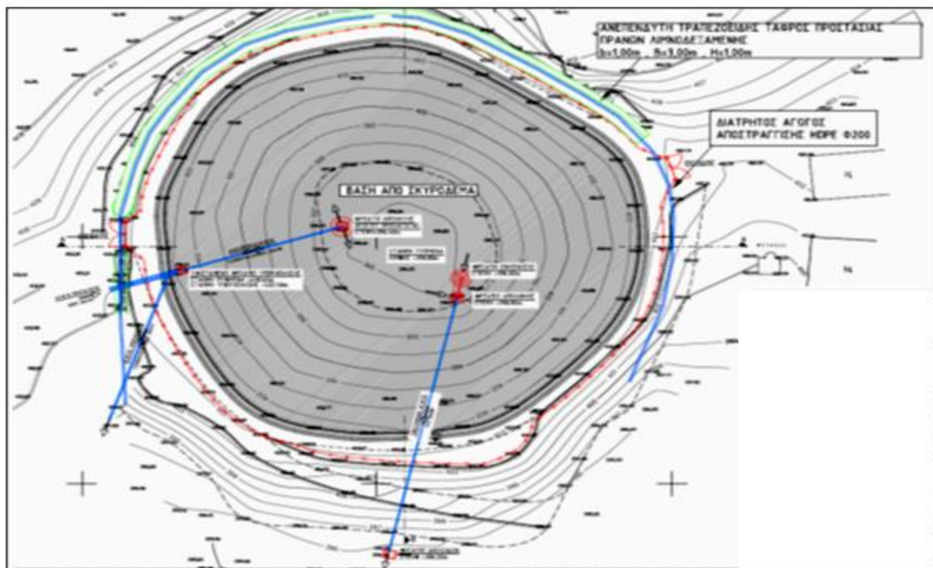
Σχέδιο 4 (απόδοση χωρίς κλίμακα) : Προτεινόμενη διαμόρφωση έργου (υδραυλικές κατασκευές και περίφραξη λιμνοδεξαμενής).
