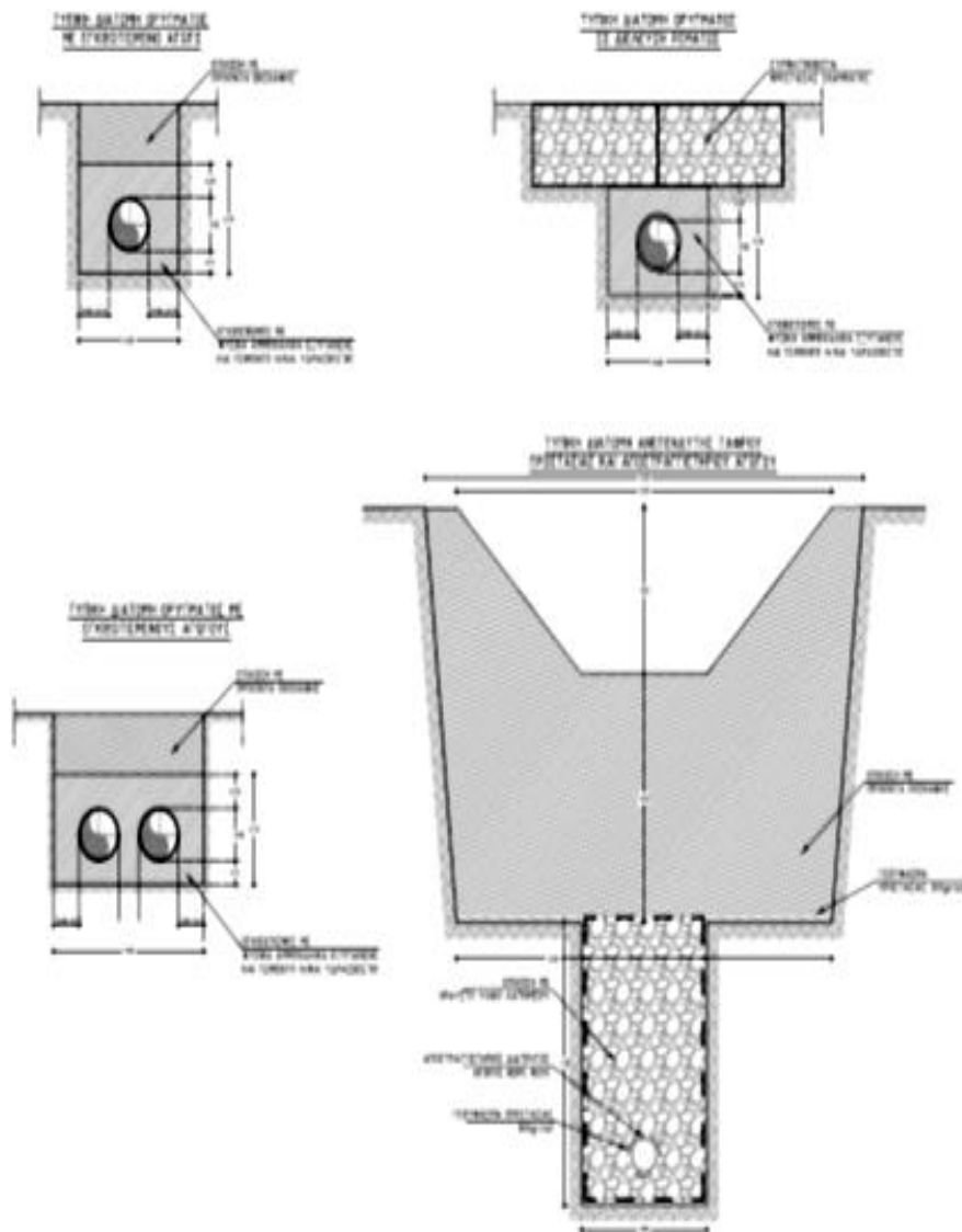
Σχέδιο 7 (απόδοση χωρίς κλίμακα) : Προτεινόμενη διαμόρφωση έργου (Τυπικές διατομές ορύγματος αγωγού/ων προσαγωγής, αποστραγγιστήριο αγωγού)
