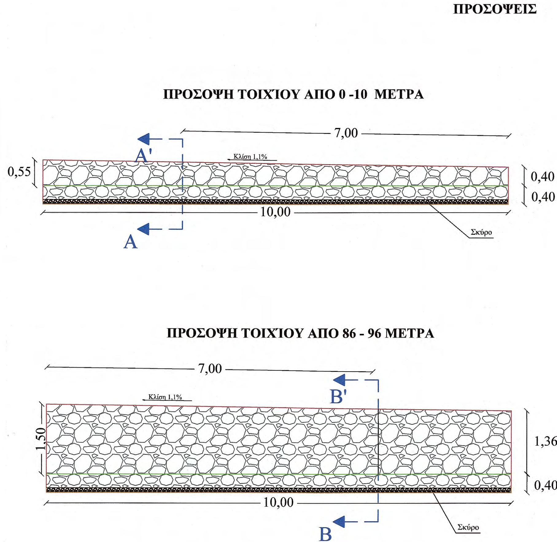
ΠΡΟΣΟΨΗ ΣΤΟ ΧΩΡΟ ΤΩΝ ΤΡΑΠΕΖΟΠΑΓΚΩΝ
