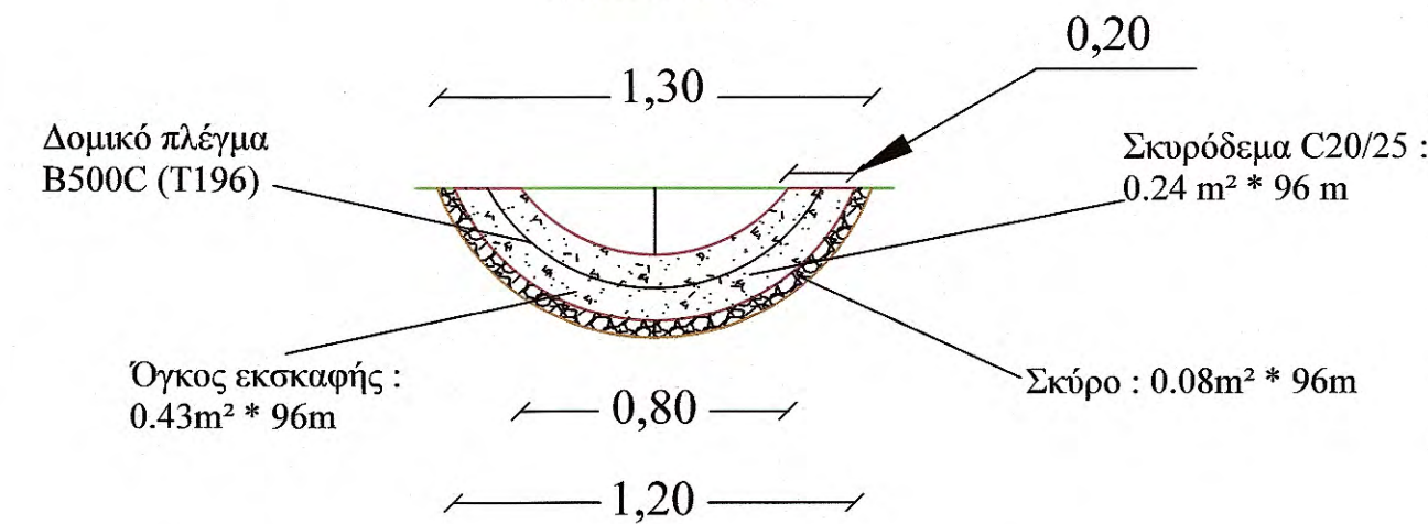
ΤΥΠΙΚΗ ΔΙΑΤΟΜΗ ΕΚΣΚΑΦΗΣ ΤΑΦΡΟΥ
