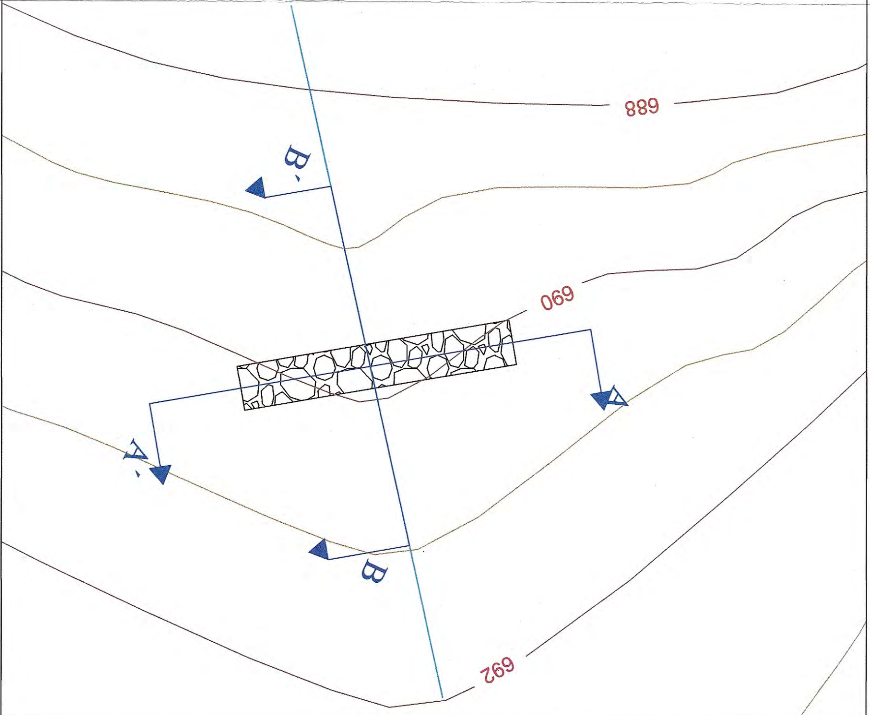
ΤΟΠΟΓΡΑΦΙΚΟ ΔΙΑΓΡΑΜΜΑ
