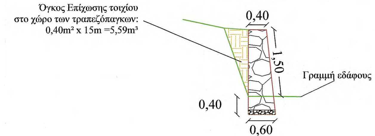
ΤΟΜΗ Γ - Γ'
