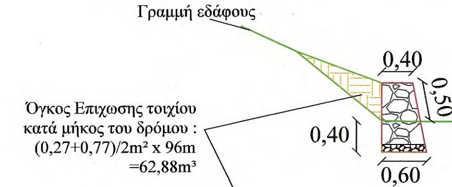
ΤΟΜΗ Α - Α'
