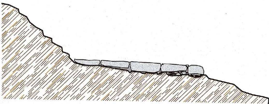
ΕΝΔΕΙΚΤΙΚΗ ΤΟΜΗ
