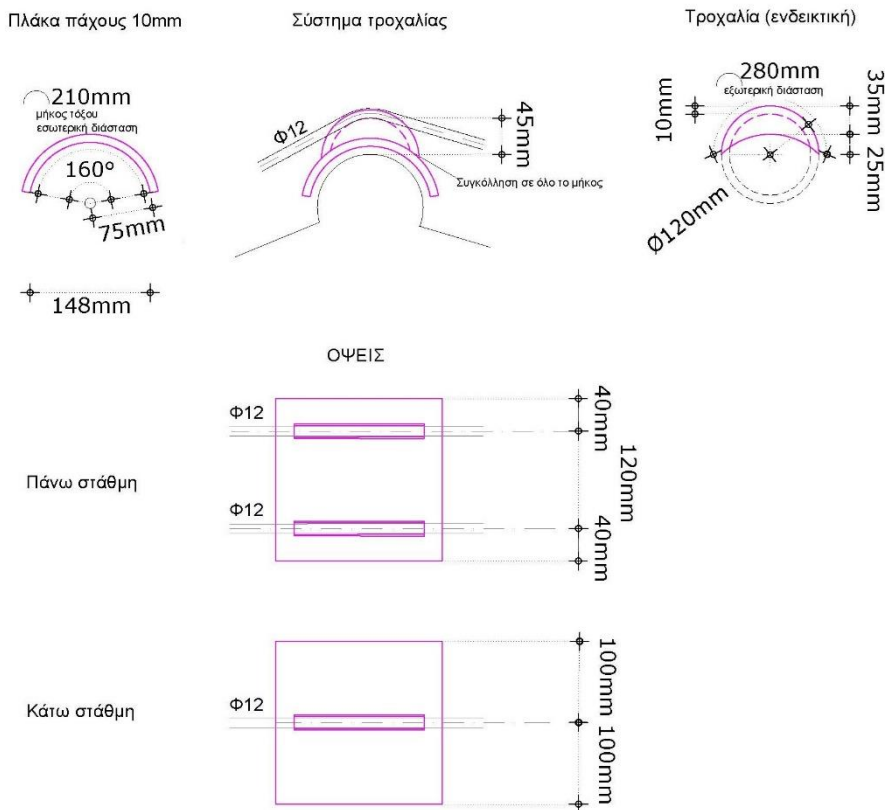
Εικόνα 3. Λεπτομέρεια πλάκας αγκύρωσης τρούλων Λιτής
