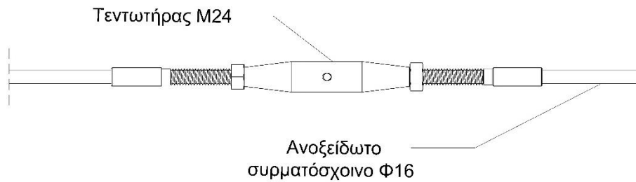
Εικόνα 6. Ενδεικτική διάταξη τεντωτήρα για σурματόσχοινο Φ16
