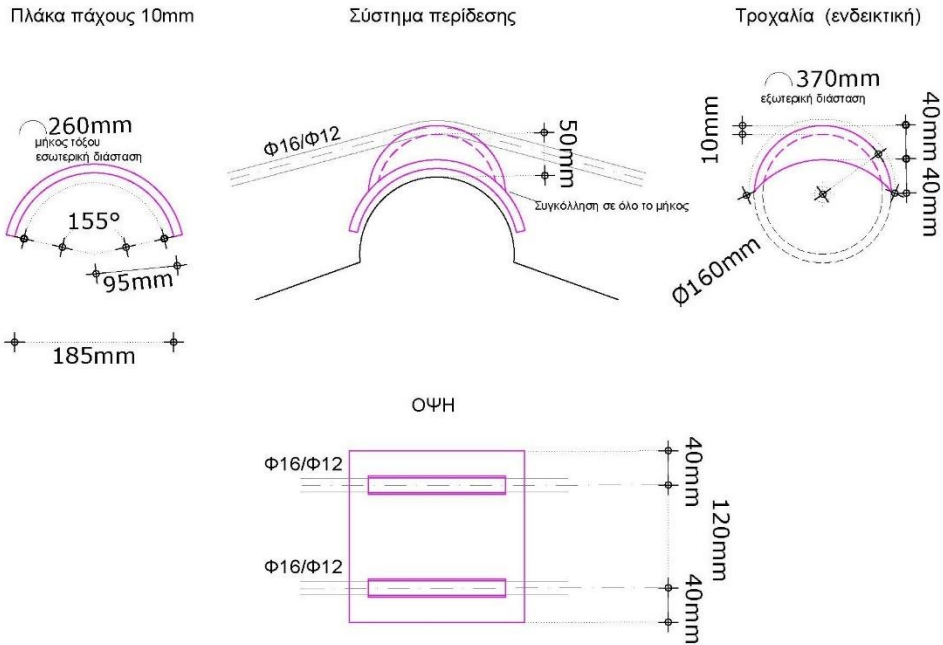
Εικόνα 4. Λεπτομέρεια πλάκας αγκύρωσης τρούλου Κυρίως Ναού
