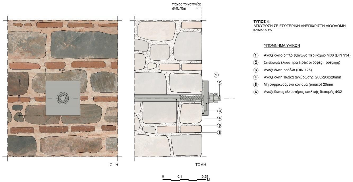
Εικόνα 1. Λεπτομέρεια πλάκας αγκύρωσης ελκυστήρων
