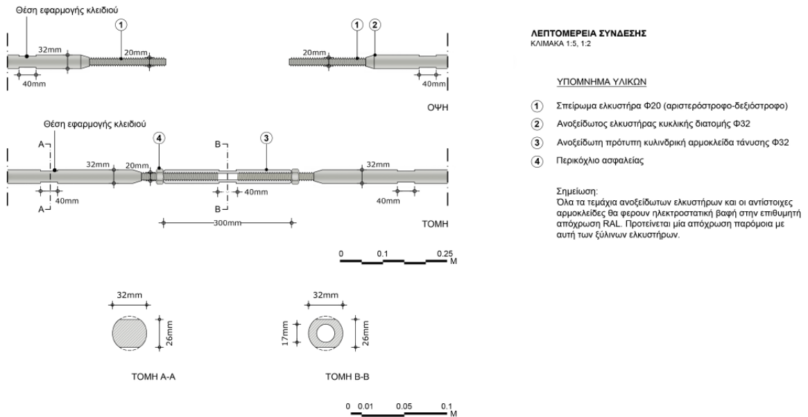
Εικόνα 2. Λεπτομέρεια σύνδεσης ελκυστήρων (αρμοκλειδες)
