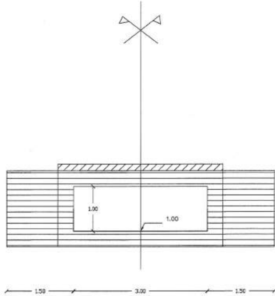
ΟΨΗ ΑΝΑΝΤΗ ΚΛ. 1:50
