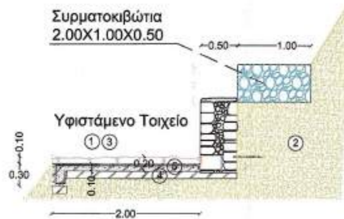
ΤΟΜΗ Α-Α'
