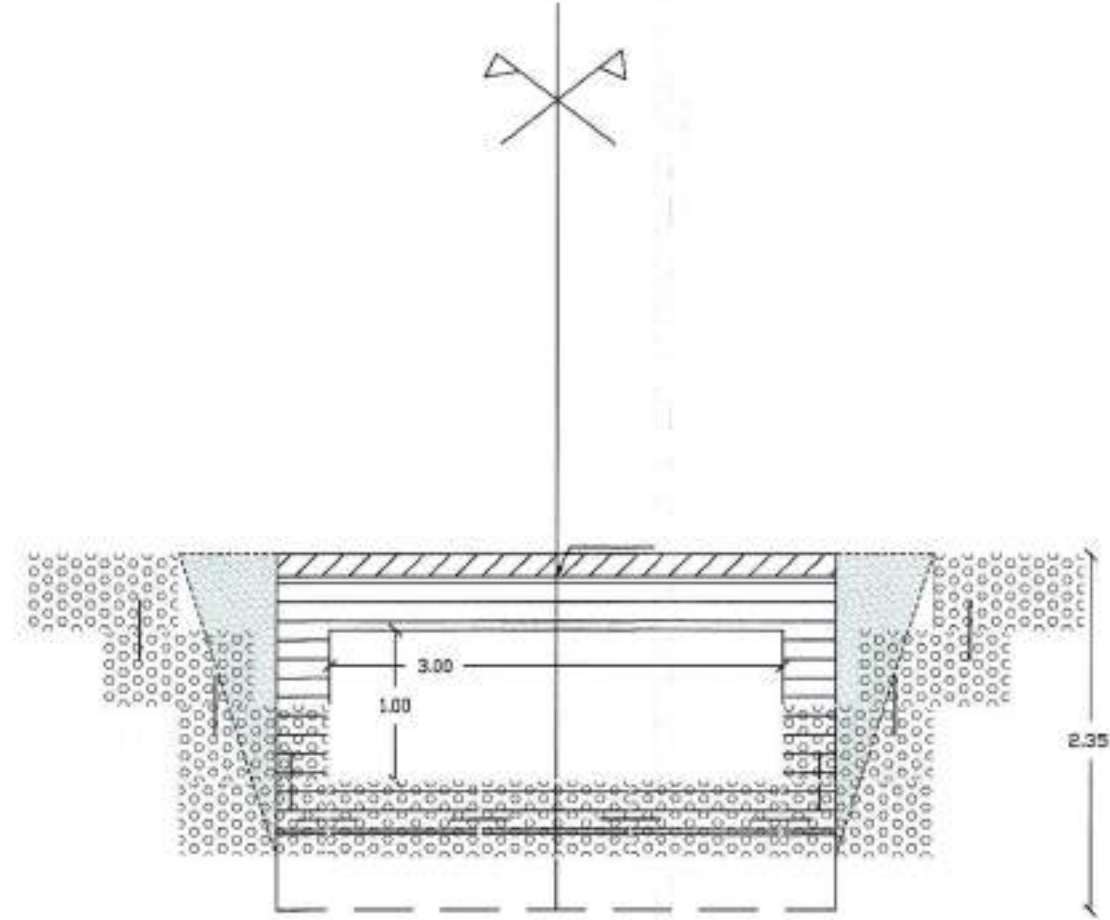
ΟΨΗ ΑΝΑΝΤΗ ΚΛ. 1:50
