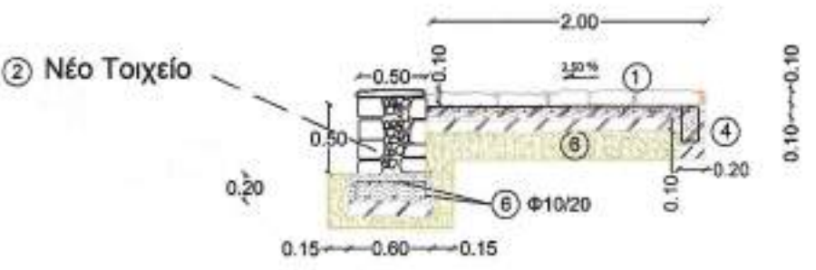
ΤΟΜΗ Β-Β'
