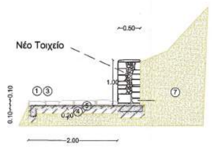
ΤΟΜΗ Α-Α'
