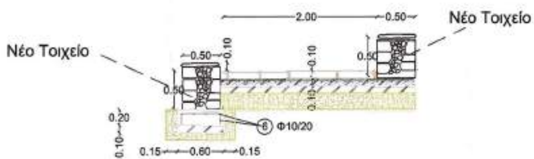
ΤΟΜΗ Α-Α'
