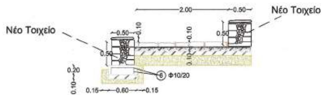
ΤΟΜΗ Α-Α'
