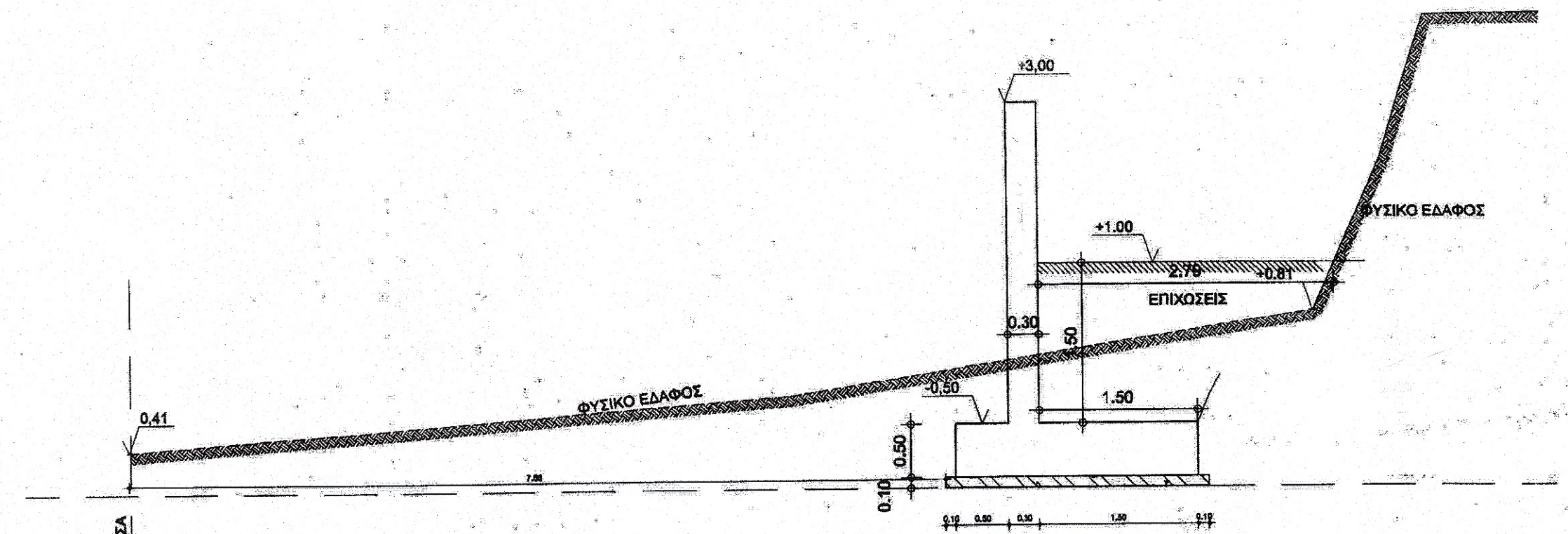
ΤΟΜΗ ΣΤΟ 25ο μ. ΤΟΙΧΕΙΟΥ
