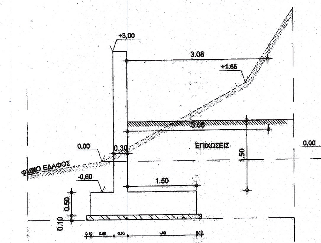
ΤΟΜΗ ΣΤΟ 40ο μ. ΤΟΙΧΕΙΟΥ
