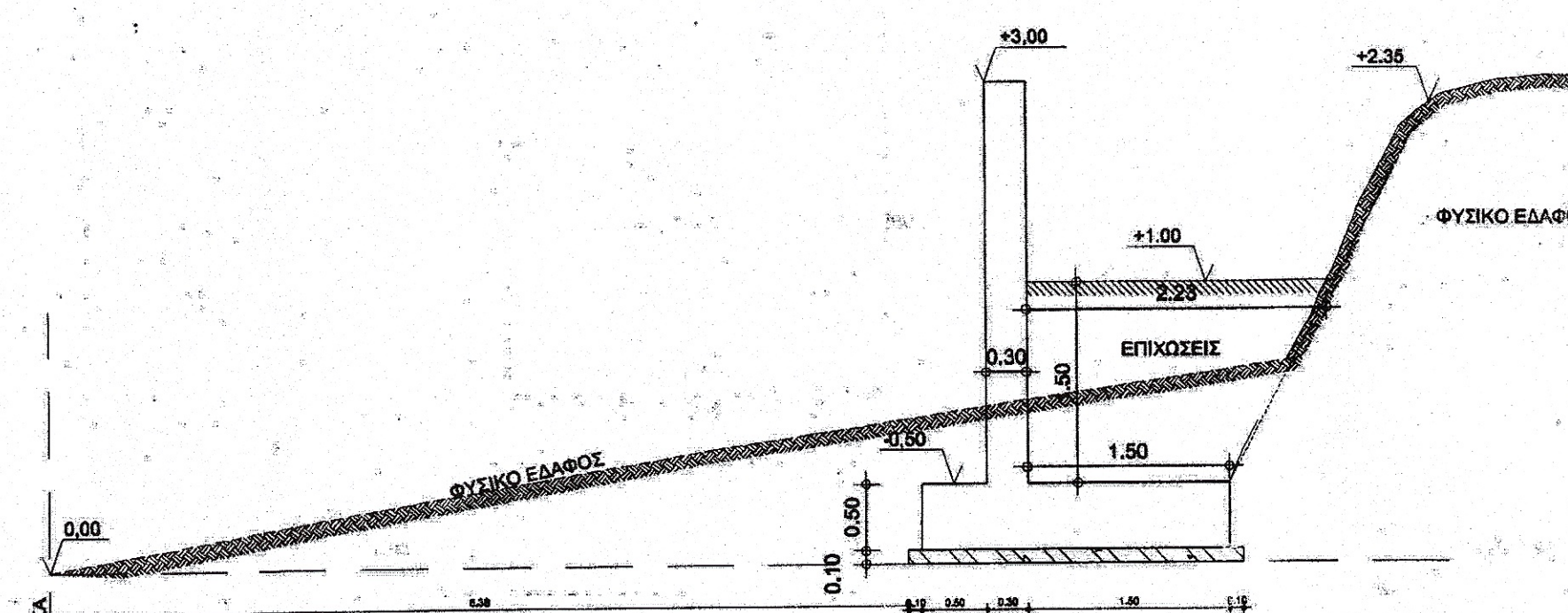
ΤΟΜΗ ΣΤΟ 10ο μ. ΤΟΙΧΕΙΟΥ
